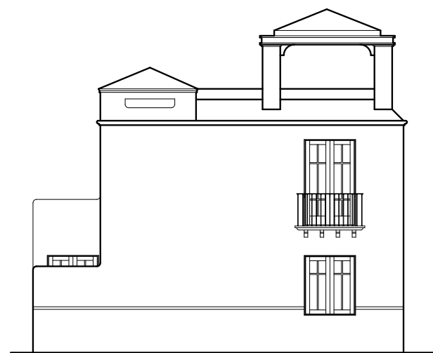
ELEVATION 2
